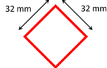
Mynd 1: Myndin sýnir hvernig mæla skal stærð merkis í samræmi við upplýsingar í töflu 1. Málín á myndinni eiga við ílát að rúmmáli 50 til 500 lítra.
