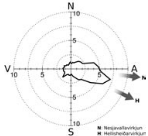
Brennisteinsvetni á Grensásvegi árið 2006 meðalstyrkur (µg/m 3 ) í ólíkum vindáttum.
