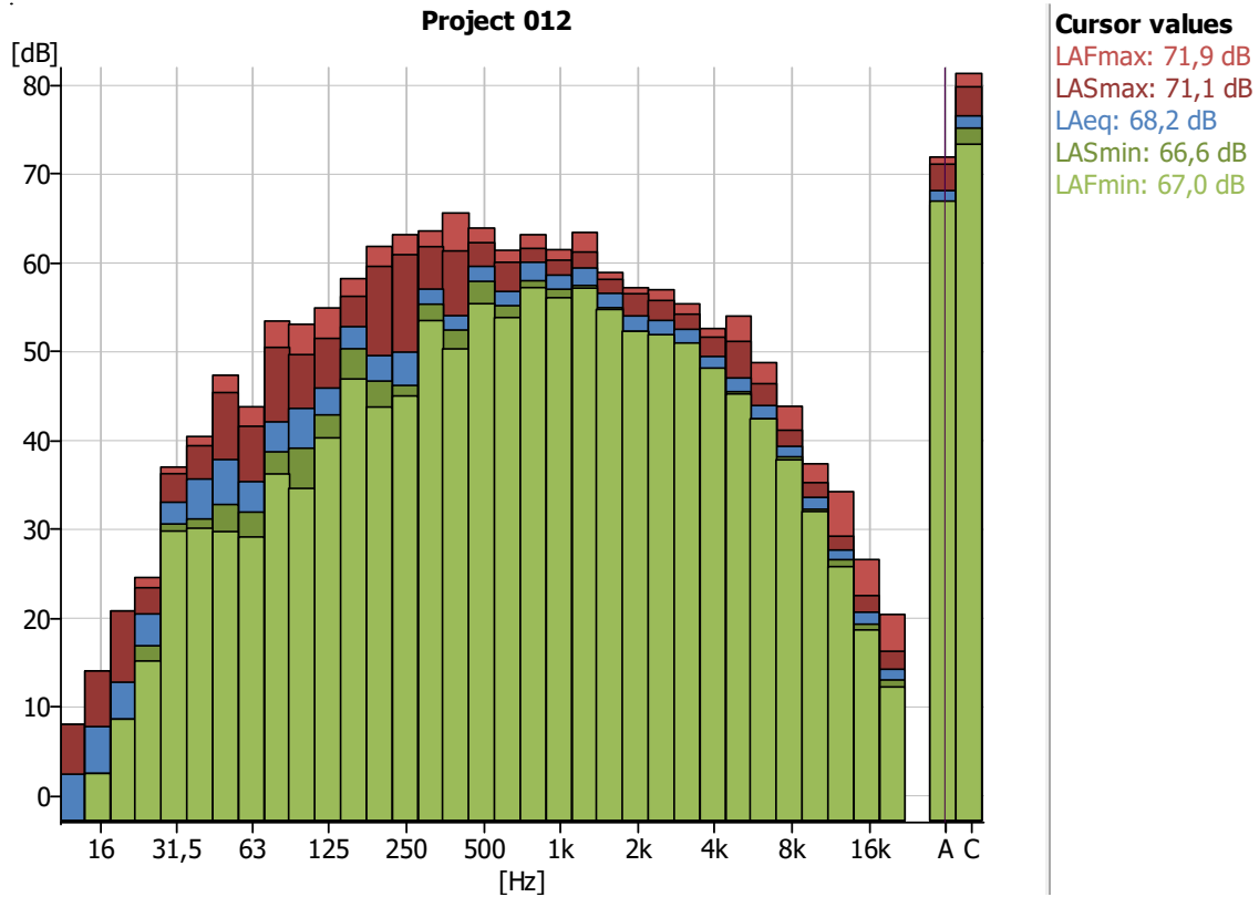
Mynd 7: Mælipunktur 11, tíðniróf ásamt hæsta og lægsta mæligildi. Engir ríkjandi tónar eru merkjanlegir í mælingu.
