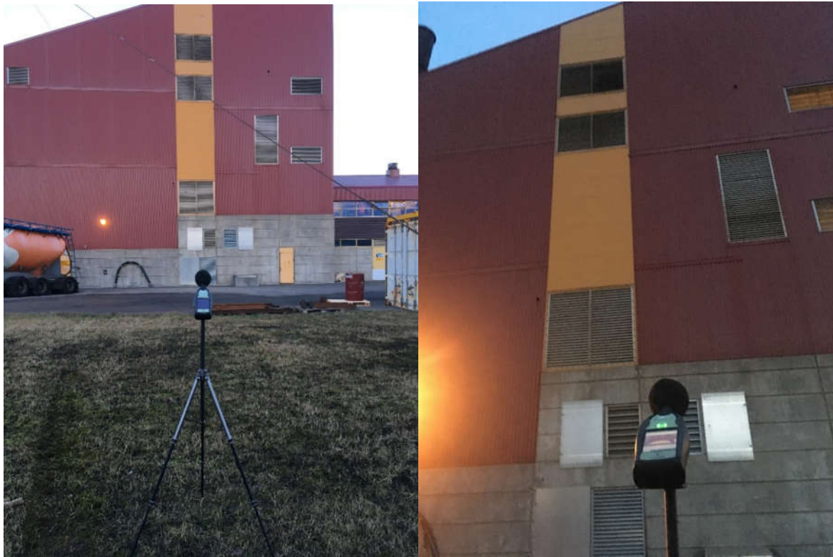
Mynd 6: Mæling nr. 2 og mæling nr. 11 við loftristar á ofnhúsi þar sem einna helst mætti vænta hávaða frá verksmiðjunni.
