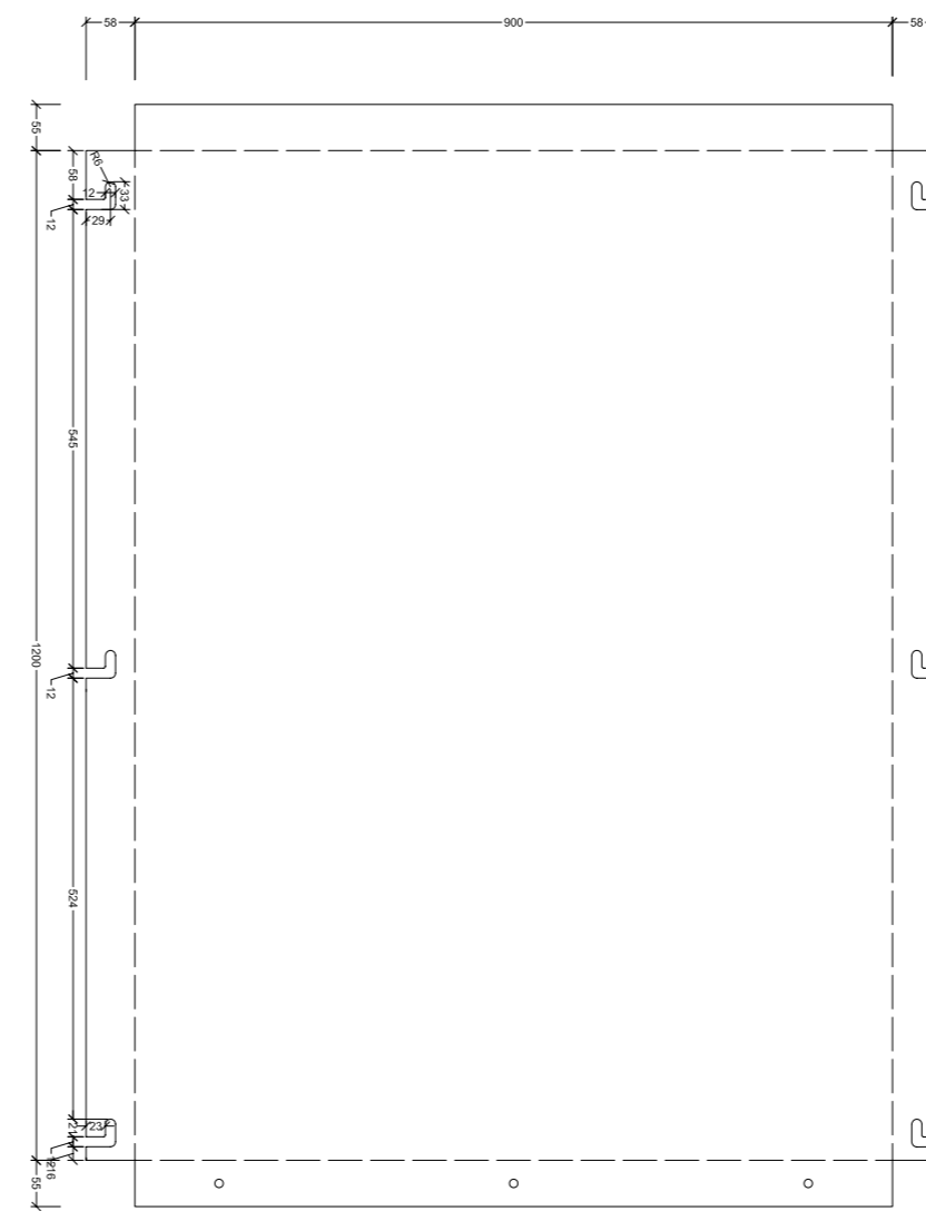
Skiltaflötur 900 x 340 mm – Aðalplata
