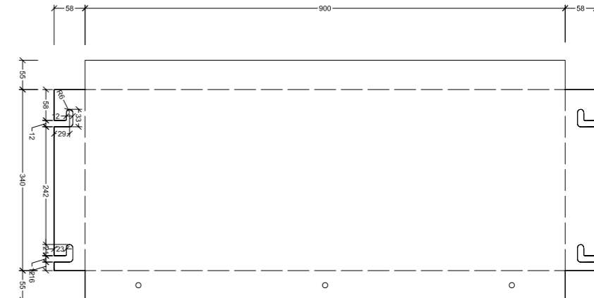
Skiltaflötur 900 x 340 mm – Aðalplata
