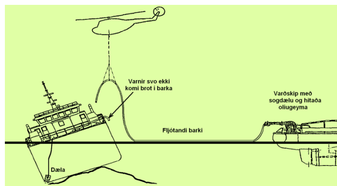
MYND 5 DÆLING ÚR STRÖNDUÐU SKIPI
