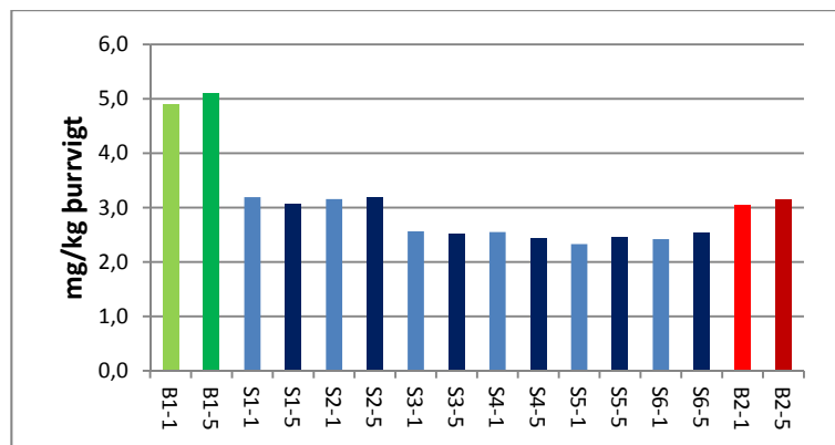
Mynd 15. Selen í mjúkvöðva krækings
