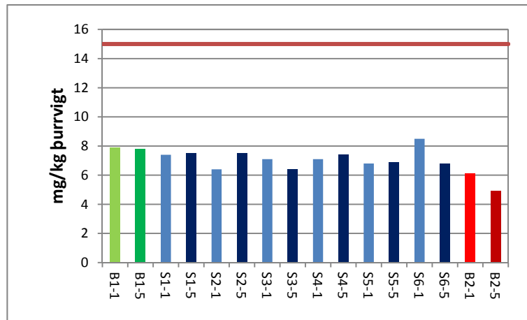
Mynd 14. Flúor í mjúkvöðva krækings
