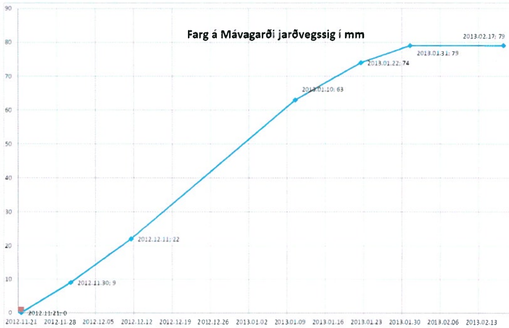
Mynd 1: Sigmælingar á fergingu
