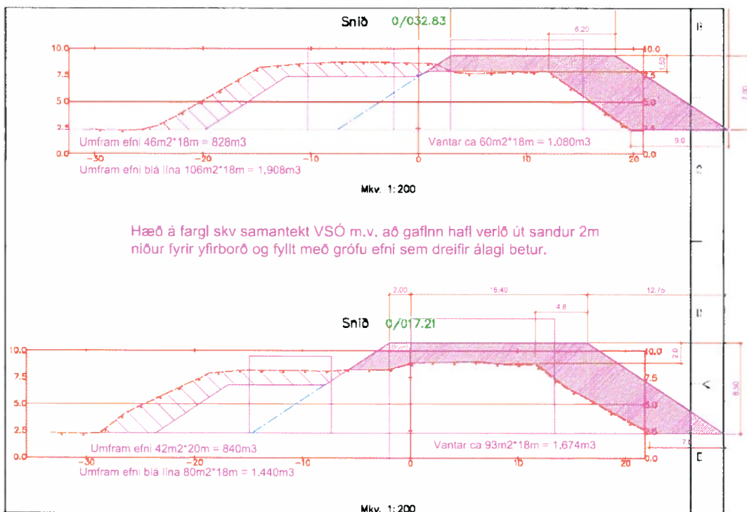
Mynd 2: Snið í farg á Mávagarði
